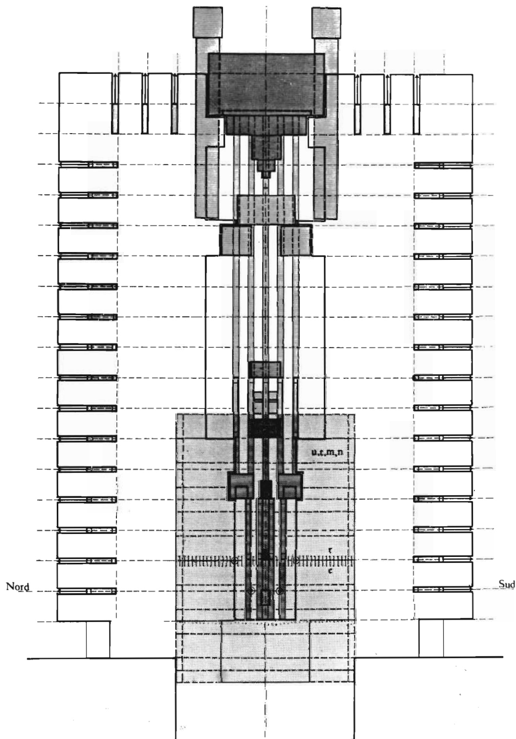
Pl. XLII les colonnes et les manteaux
